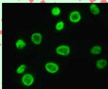
Senescence Marker Antibody Panel (#ARG30340)に含まれる抗体(抗p21, Rabbit-Poly)を用いた免疫細胞染色像 試料: HeLa細胞 抗体希釈倍率: 1:100
