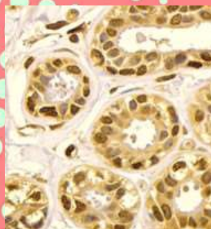
CAF Marker Antibody Panel (#ARG30347)に含まれる抗体(抗S100A4, Rabbit-Poly)を用いた免疫組織染色像 試料: パラフィン包埋ヒト乳房 抗体希釈倍率: 1:100
